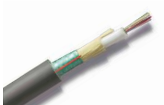
CABLE MONOTUBO
